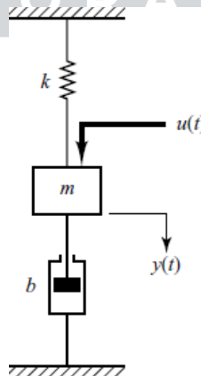
Gambar 3. 21 Parameter Sistem Pegas Massa
