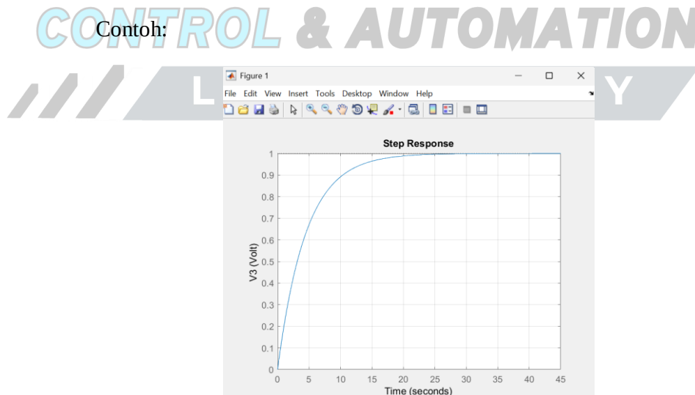
Gambar 2. 2 Respons Unit Step Sistem Orde Satu.
