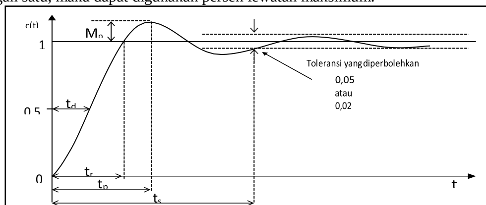
Gambar 3. 7 Kurva Respons Sistem Orde Dua Underdamped dengan Masukan Unit Step
