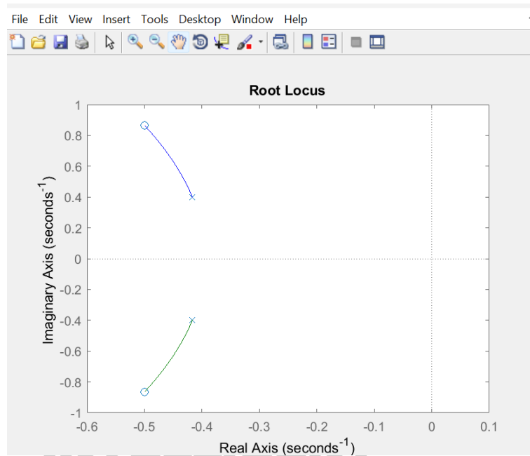
Gambar 4. 5 Poles Dan Zero Berpasangan
