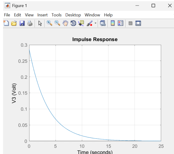
Gambar 2. 3 Respons Unit Impulse Sistem Orde Satu.
