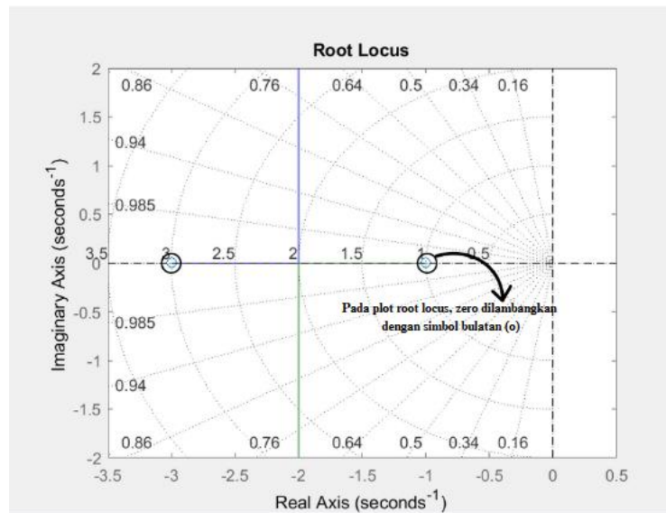
Gambar 4. 2 Bentuk Kurva zero Root Locus
