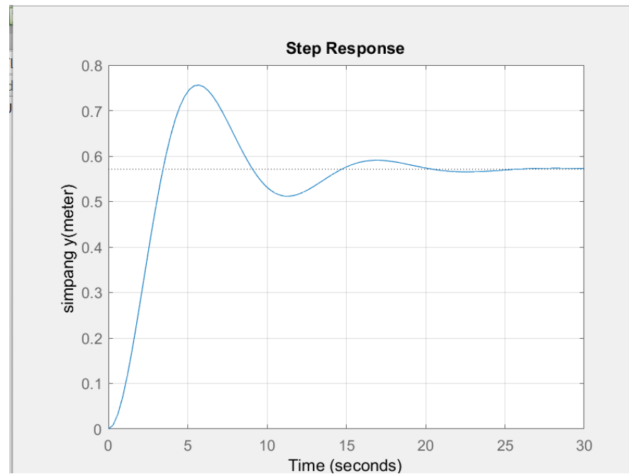
Gambar 3. 2 Kurva Keluaran Step Sistem Orde 2
