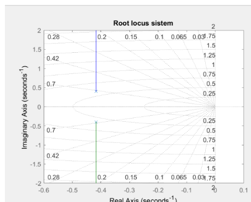
Gambar 4. 4 Simetris terhadap sumbu real
