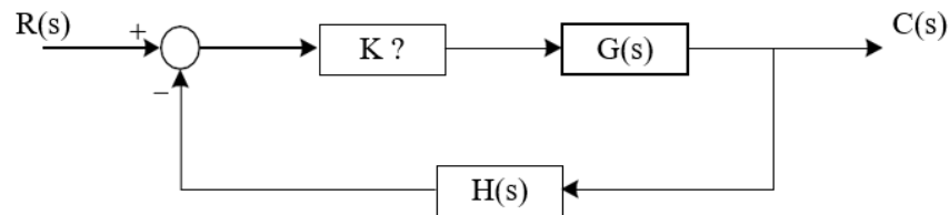
Gambar 4. 3 Sistem Loop Tertutup
