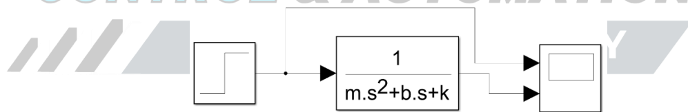
Gambar 3. 9 Diagram Blok Sistem Orde 2
