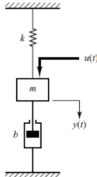
Gambar 4. 16 parameter sistem pegas massa
