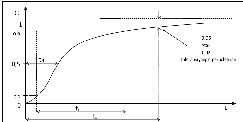
Gambar 3. 8 Kurva Respon Sistem Orde Dua Overdamped dengan Masukan Unit Step
