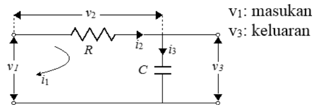
Gambar 2. 5 Rangkaian RC seri
