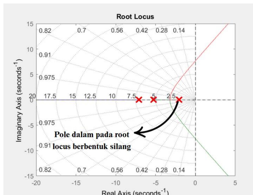
Gambar 4. 1 Bentuk Kurva pole Root Locus
