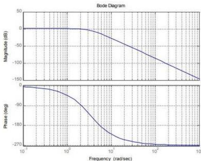
Gambar 4. 10 Diagram Bode Suatu Sistem
