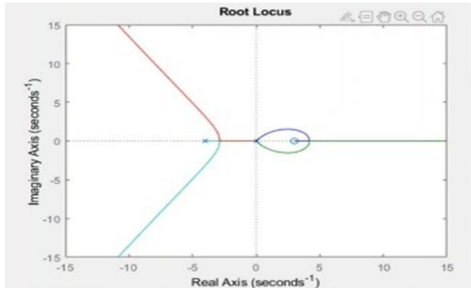
Gambar 4. 9 Kondisi Root Locus tidak Stabil
